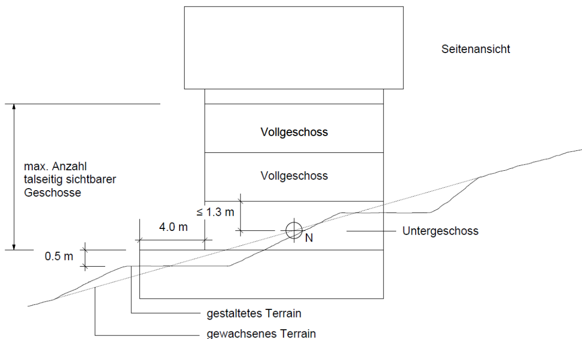
Abb. 1: Talseitig sichtbare Geschosse – Seitenansicht
