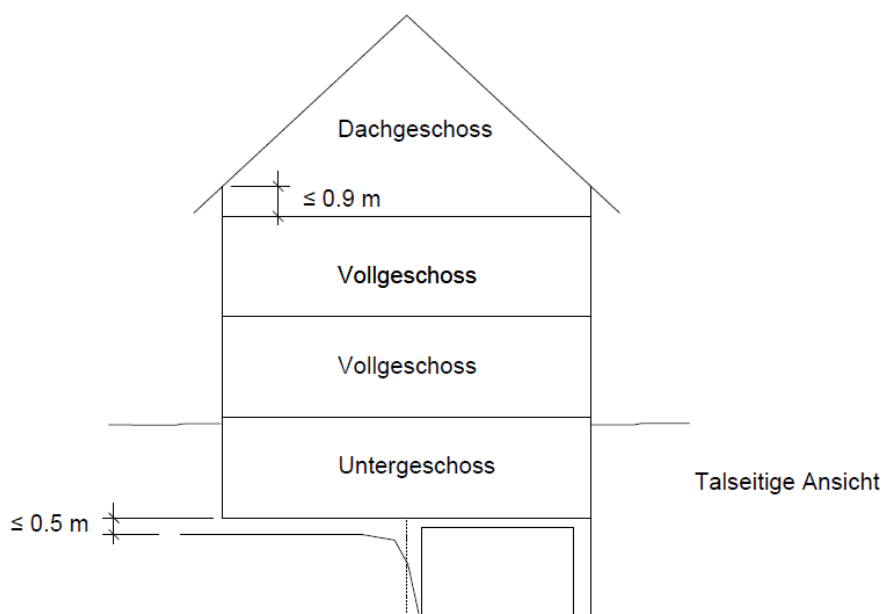
Abb. 2: Talseitig sichtbare Geschosse – Hauptansicht
